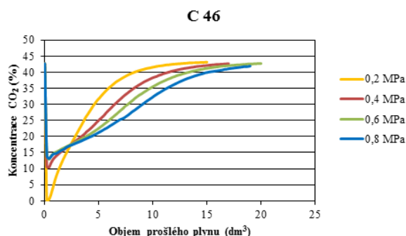
Obr. 3. Průnikové křivky pro adsorbent C 46 naměřených s použitím modelové směsi plynů v laboratorních podmínkách.
