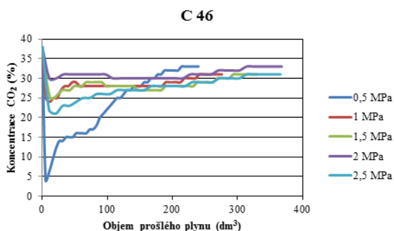
Obr. 7. Průnikové křivky pro adsorbent C 46 naměřené s použitím reálného bioplynu za vyšších tlaků.
