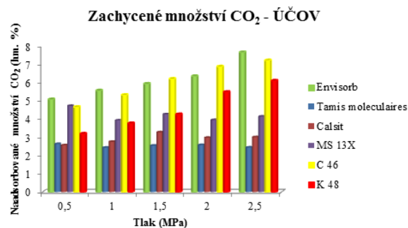
Obr. 8. Měření adsorbovaného množství CO 2 pro jednotlivé adsorbenty při různých tlacích s použitím reálného bioplynu.
