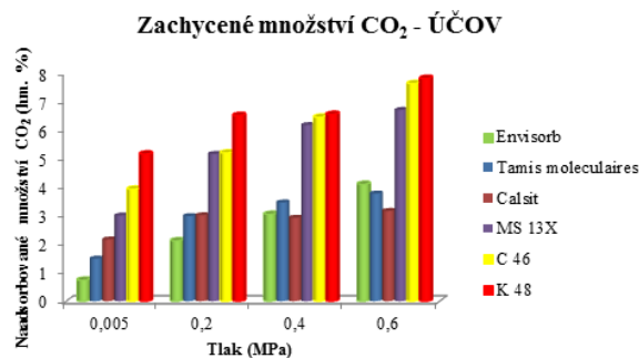
Obr. 6. Měření adsorbovaného množství CO 2 pro jednotlivé adsorbenty při různých tlacích s použitím reálného bioplynu.
