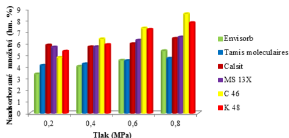
Obr. 4. Měření adsorbovaného množství CO 2 pro jednotlivé adsorbenty při různých tlacích v laboratorních podmínkách s použitím modelového plynu.
